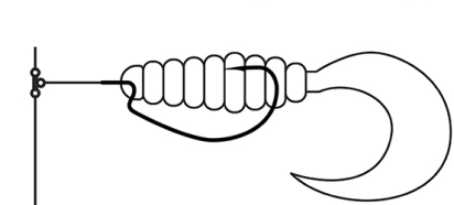
Оснастка с отводным поводком
