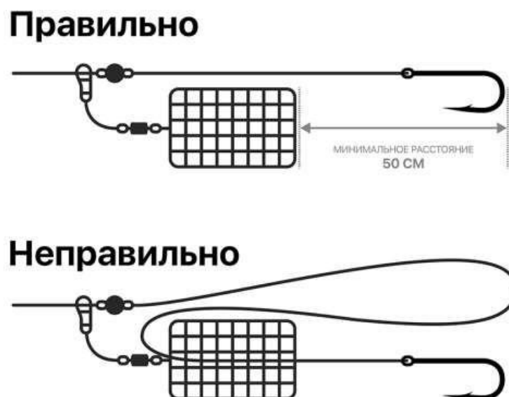
Рис. 3. Длина поводка
