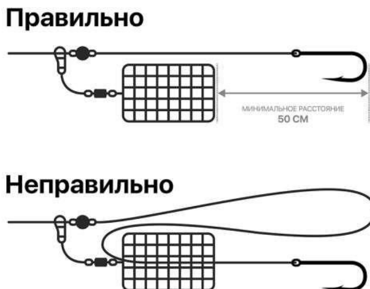
Рис. 3. Длина поводка
